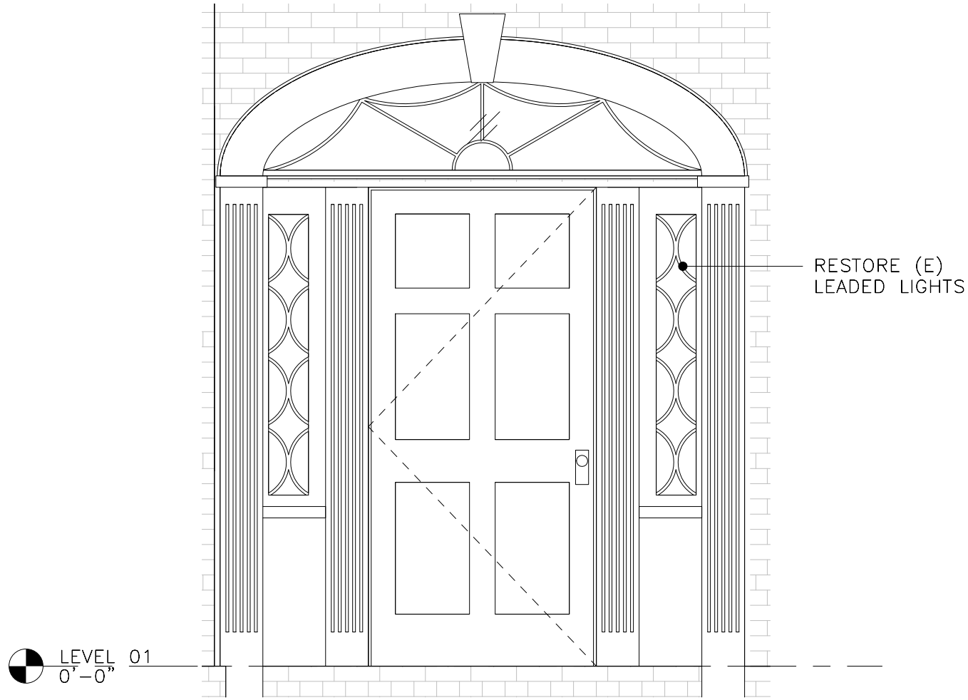
5 FAN & SIDE LIGHTS AT FRONT DOOR
